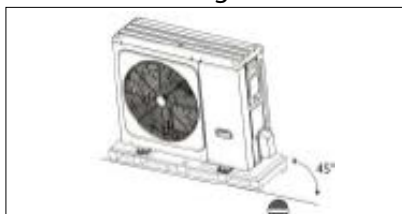
3/4. Luta inte aggregatet mer än 45° och lägg det inte ner sidledes
