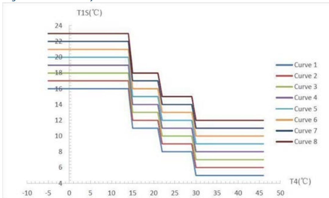
Låga klimatkurvor för kyl drift
