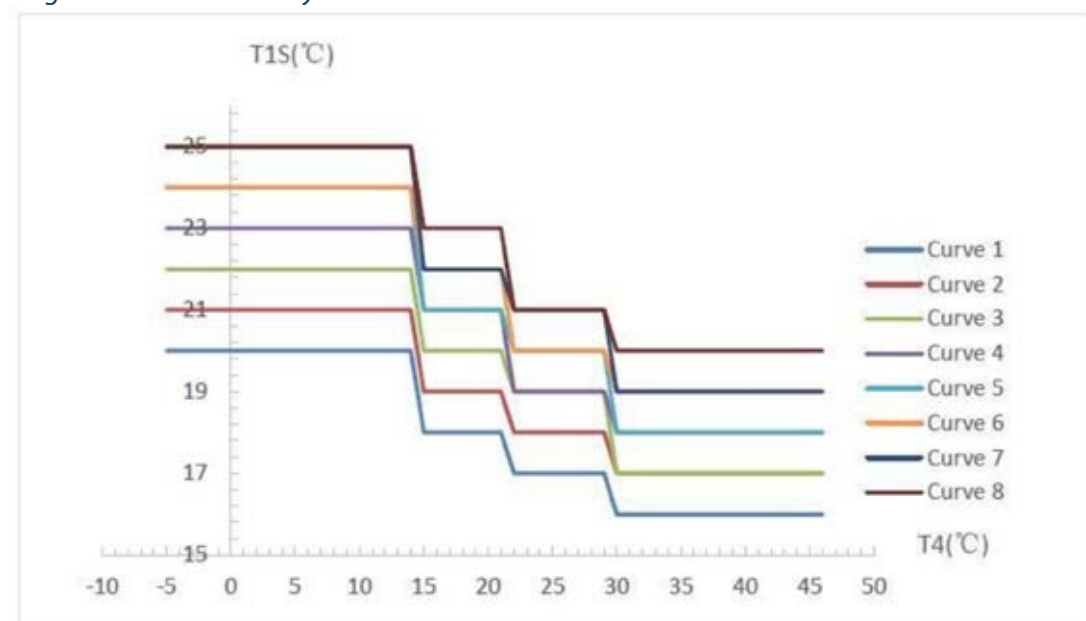
Höga klimatkurvor för kyl drift
