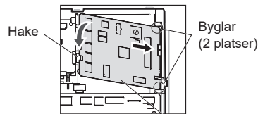
Extern ingångs-/utgångskrets kort
